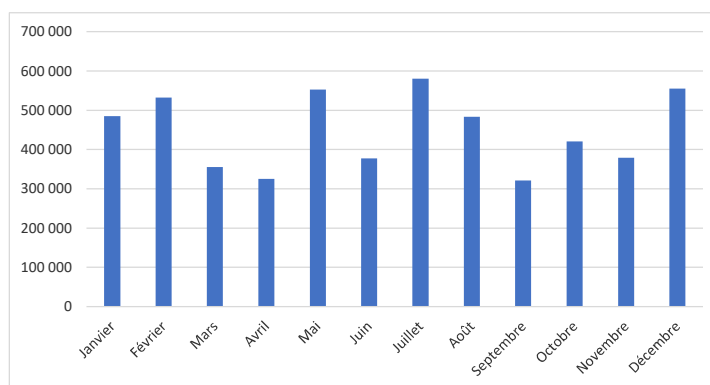
Volume mensuel entrant à la station d'épuration de Givors en 2021 (en m³)
