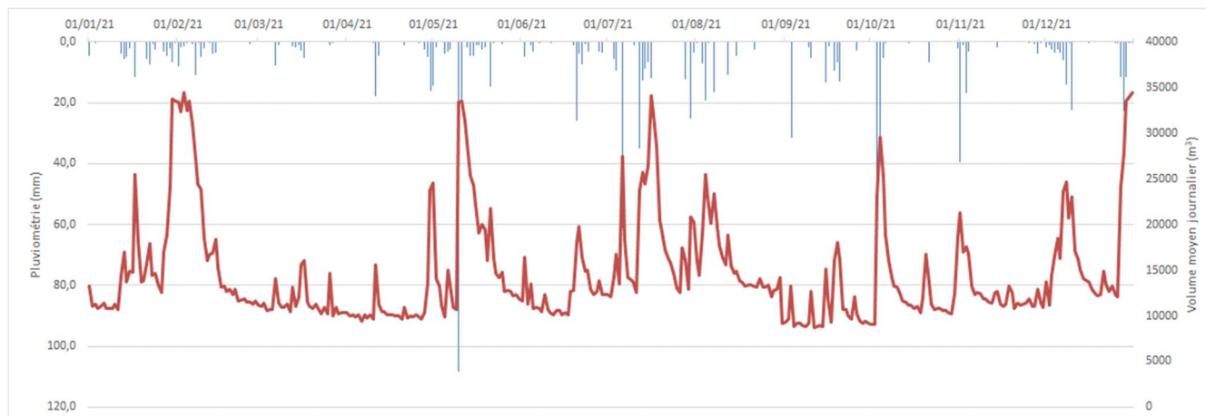
Corrélation entre pluviométrie journalière et volume moyen journalier entrant à la station d'épuration de Givors
